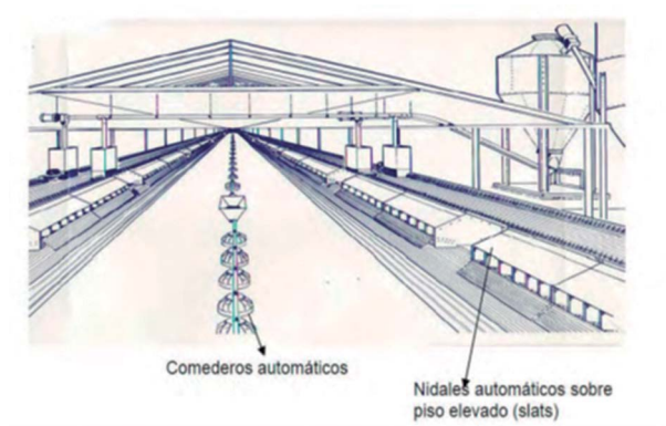
Figura 89: Disposición de los equipos para producción a piso
