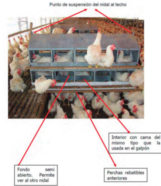
Figura 90: Disposición de nidales en el galpón
