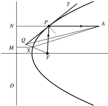
Figura 8.5 Reflexión en una parábola.
