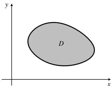
Figura 15.11 Un dominio simplemente conexo.
