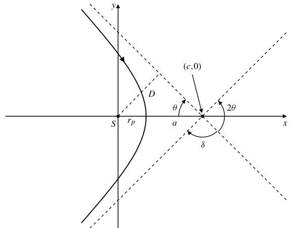
Figura 11.27 Trayectoria de un meteoro.
