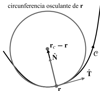
Figura 11.16 Circunferencia osculante.
