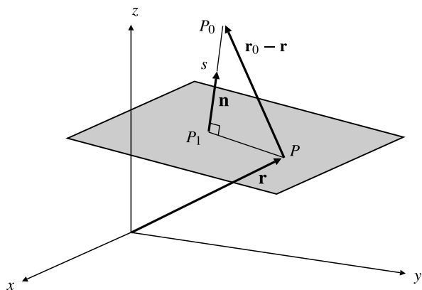
Figura 10.32 La distancia de P_0 al plano \mathcal{P} es la longitud del vector proyección de \overline{PP_0} sobre el vector normal \mathbf{n} al plano \mathcal{P} , siendo P un punto cualquiera de \mathcal{P} .
