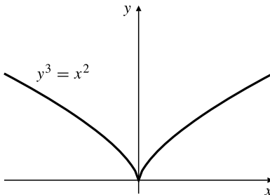
Figura 13.16 El mínimo de y se produce en un punto de la curva donde ésta no tiene tangente.
