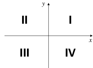
Figura P.10 Los cuatro cuadrantes.
