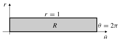
Figura 14.27 El dominio en el plano r\theta .
