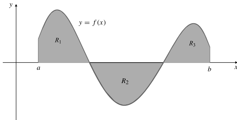
Figura 5.12 \int_a^b f(x) dx es igual al área R_1 - \text{área } R_2 + \text{área } R_3 .
