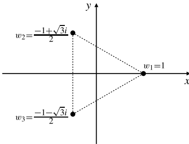
Figura I.8 Las raíces cúbicas de la unidad.
