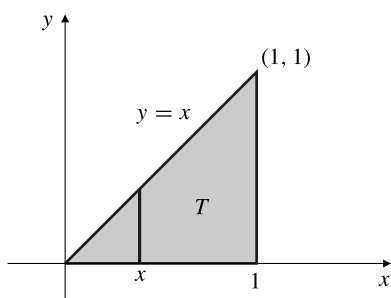
Figura 14.16 El dominio triangular T con una recta vertical que indica iteración con integral interna en la dirección de y .
