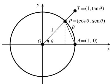
Figura 2.21 Área \triangle OAP < \text{Área sector } OAP < \text{Área } \triangle OAT .
