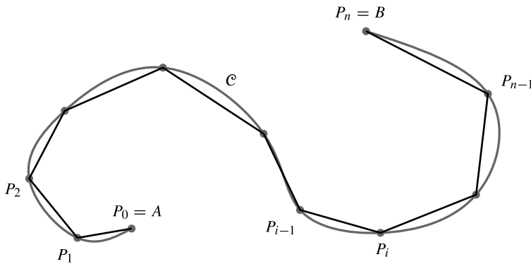
Figura 7.21 Aproximación poligonal a la curva \mathcal{C} .
