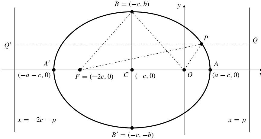
Figura 11.23 La suma de las distancias desde cualquier punto P de la elipse a los dos focos O y F es constante, y vale \varepsilon veces la distancia entre las directrices.
