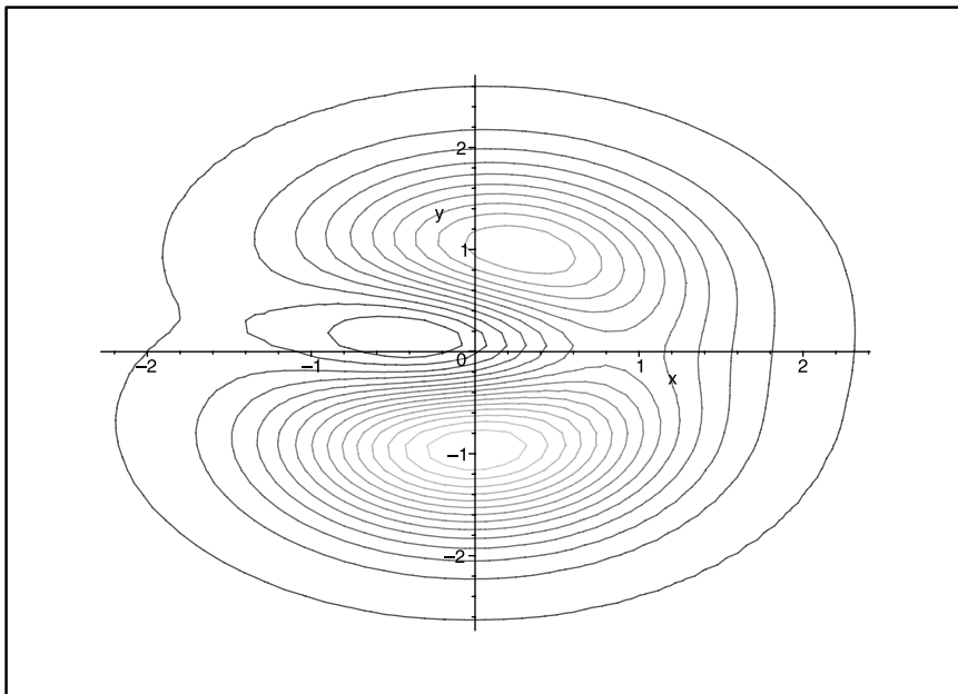
Figura 13.27 Contornos de f(x, y) en el Ejemplo 2.
