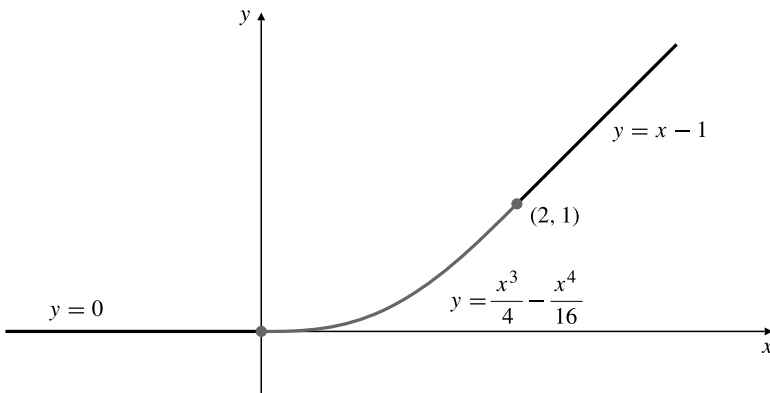
Figura 11.21 Unión de dos vías rectas mediante una vía curva.
