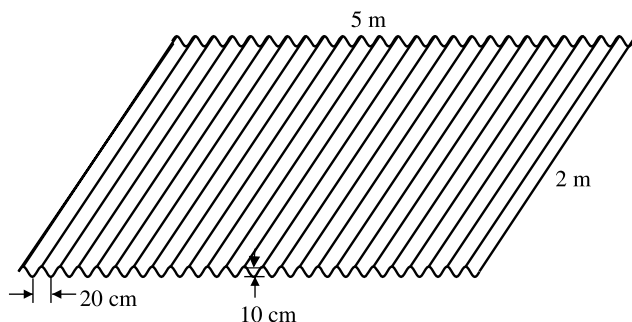
Figura 7.23 Panel ondulado para techados.
