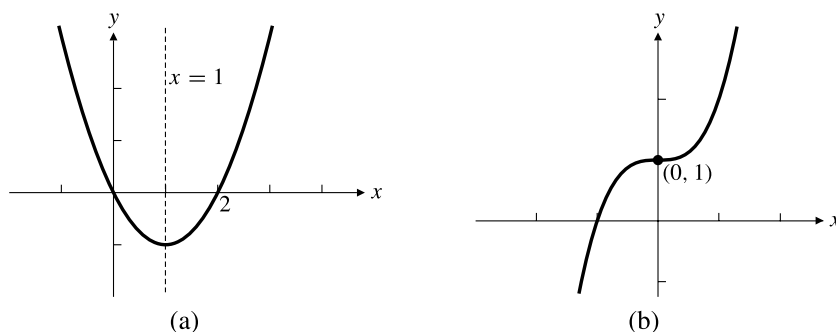
Figura P.51 (a) La gráfica de g(x) = x^2 - 2x es simétrica respecto a x = 1 . (b) La gráfica de y = h(x) = x^3 + 1 es simétrica respecto al punto (0, 1) .
