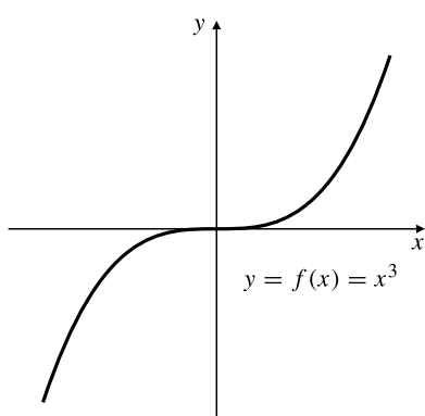
Figura 4.20 x = 0 es un punto crítico de f(x) = x^3 y f tiene un punto de inflexión en dicho punto.
