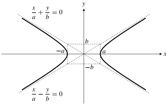
Figura P.32 La hipérbola \frac{x^2}{a^2} - \frac{y^2}{b^2} = 1 y sus asíntotas.
