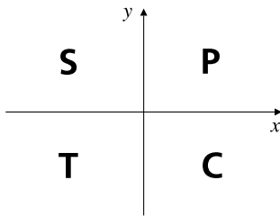
Figura P.81 La regla CPST.
