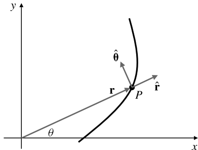
Figura 11.25 Vectores de la base en direcciones crecientes de r y \theta .
