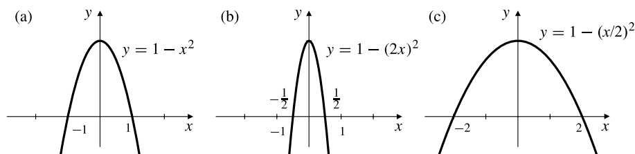
Figura P.27 Escalado horizontal:
