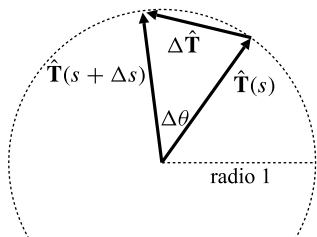
Figura 11.15 |\Delta\hat{\mathbf{T}}| \approx |\Delta\theta| para valores pequeños de |\Delta s| .
