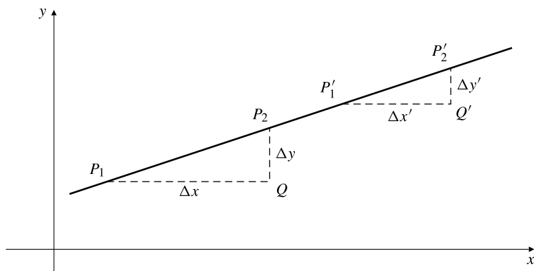
Figura P.15 \Delta y/\Delta x = \Delta y'/\Delta x' porque los triángulos P_1QP_2 y P'_1Q'P'_2 son semejantes.
