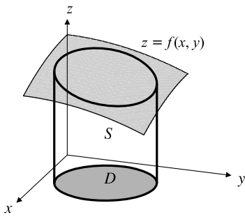
Figura 14.1 Una región sólida S dispuesta por encima del dominio D en el plano xy y por debajo de la superficie z = f(x, y) .
