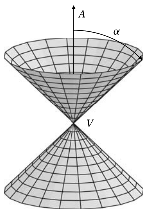
Figura 8.1 Un cono de vértice V , eje A y semiángulo vertical \alpha .
