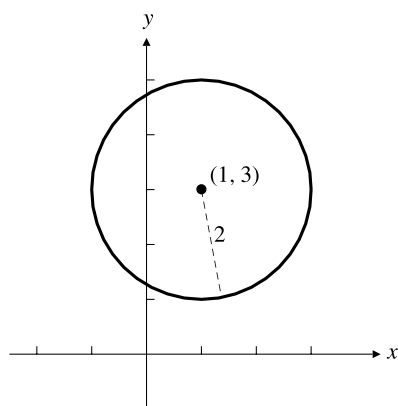
Figura P.20 La circunferencia de ecuación (x - 1)^2 + (y - 3)^2 = 4 .
