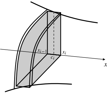
Figura 7.3 Volumen de una rodaja.
