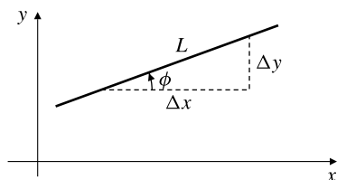
Figura P.16 La recta L tiene una inclinación de \phi .
