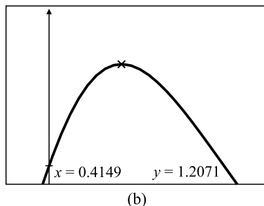
Figura 1.28 La utilización de la función «zoom» permite ampliar parte de la curva (a) cerca de su valor máximo de forma que ocupe toda la pantalla (b), manteniendo la forma de la curva.
