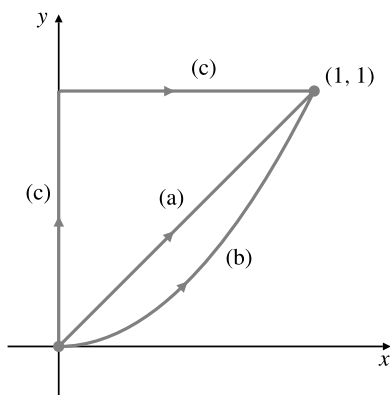
Figura 15.9 Tres caminos desde (0, 0) hasta (1, 1) .
