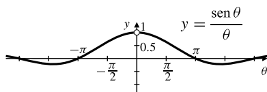
Figura 2.20 Parece que \lim_{\theta \rightarrow 0} (\text{sen } \theta)/\theta = 1 .
